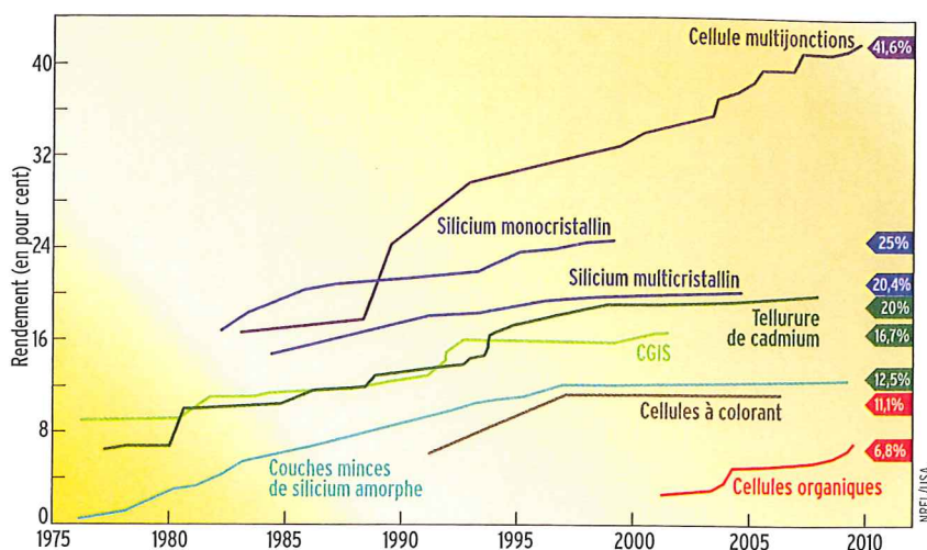
LES RENDEMENTS RECORDS en laboratoire de l'ensemble des filières photovoltaïques.
